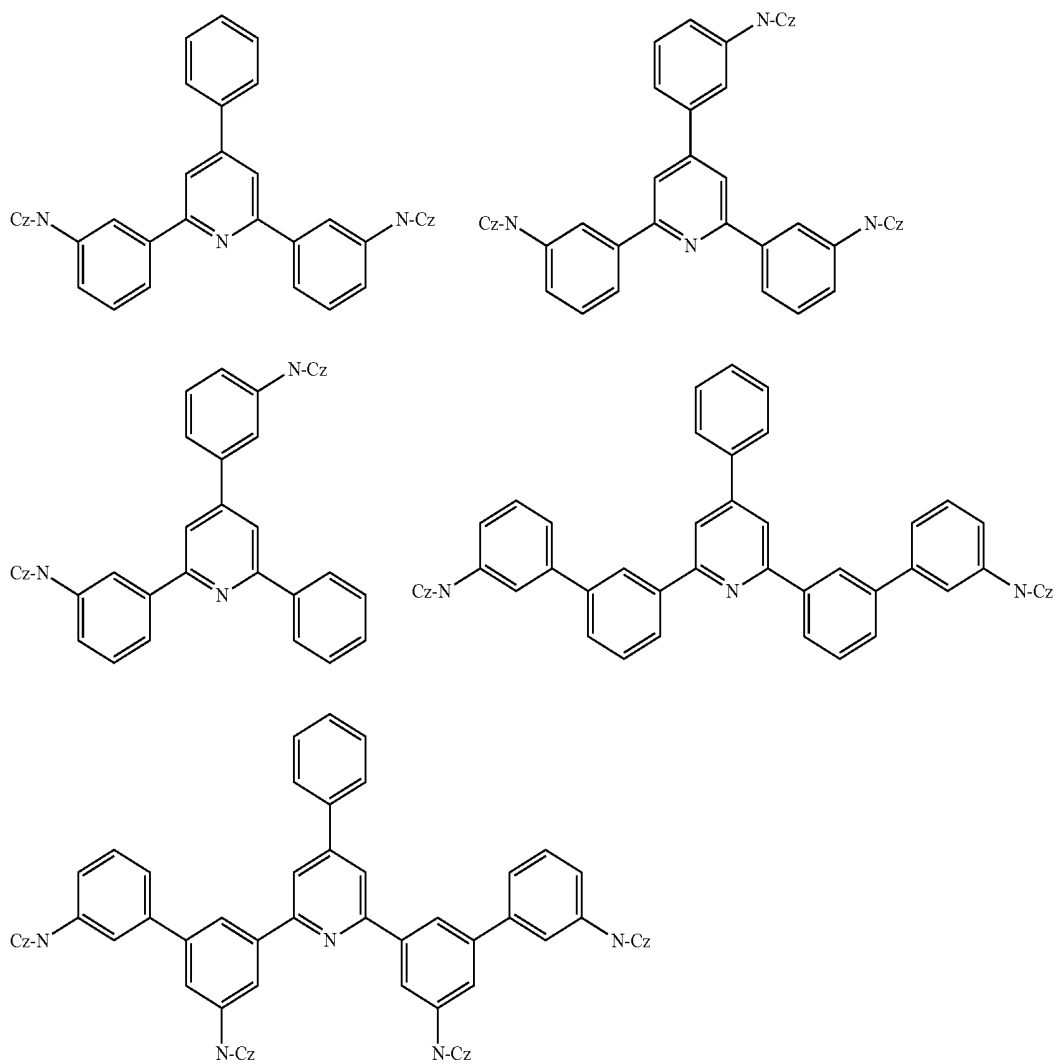
[Chem 9]
