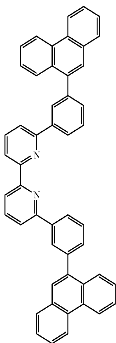
[Chem 9]
