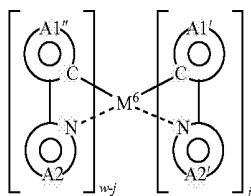
[Chem 38]
